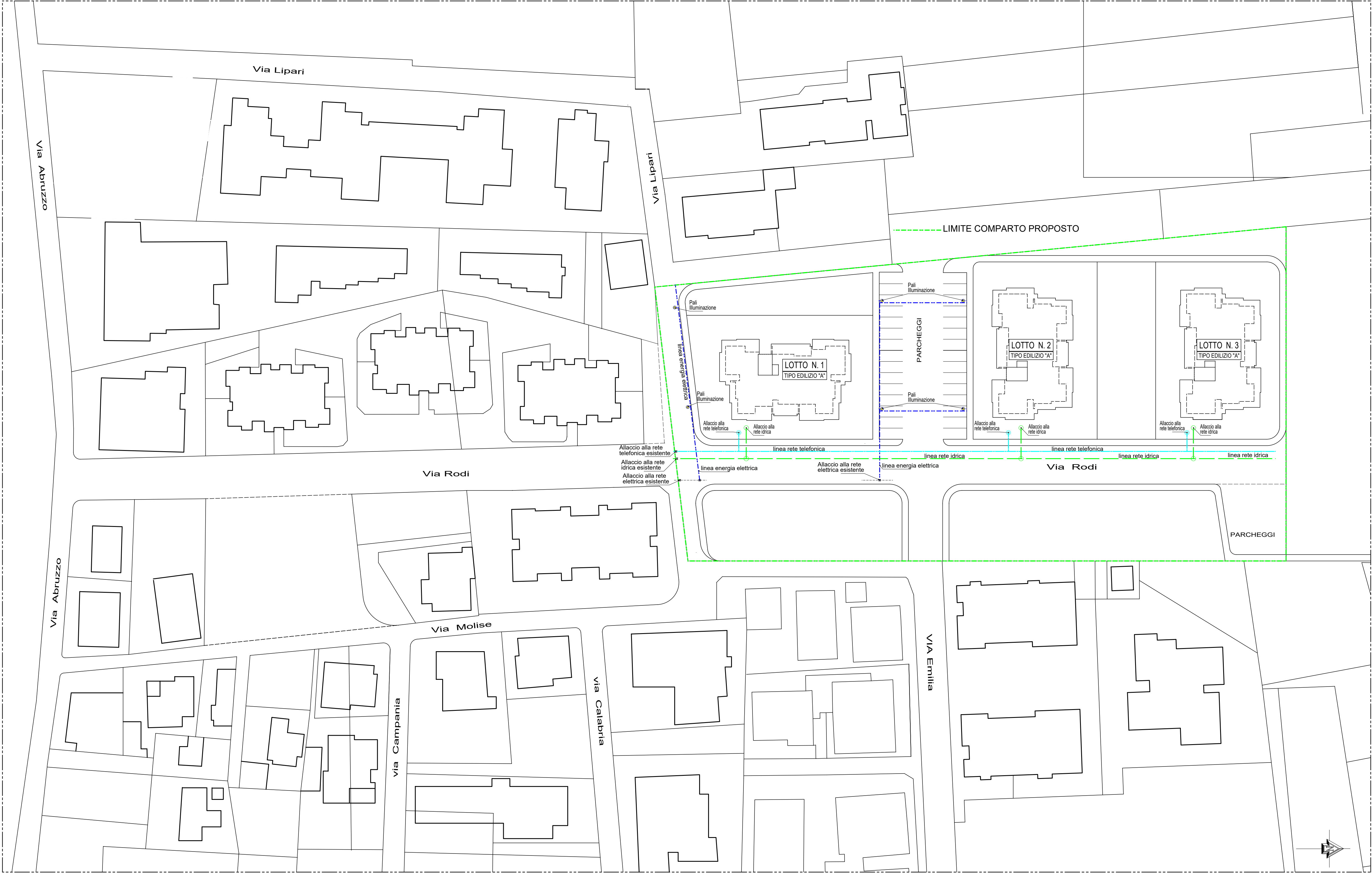
Planimetria Scala 1/500
